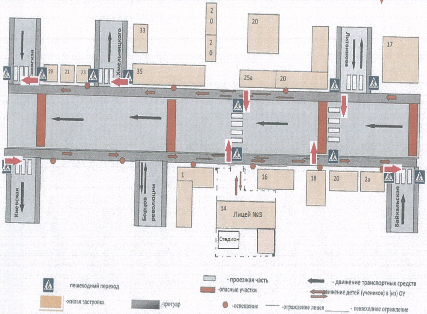
II. Схема организации дорожного движения в непосредственной близости от МБОУ г. Иркутск лицей №3 с размещением соответствующих технических средств, маршруты движения детей и расположения парковочных мест
