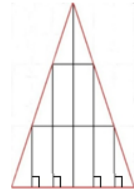
Рис. 3. Схема конструкции грани зенитного фонаря
